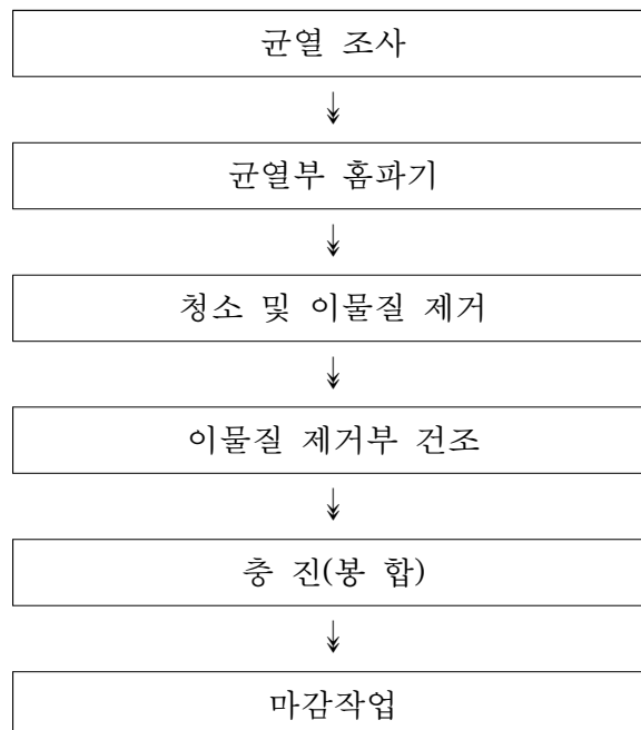
【그림 7.2.5】 아스팔트 균열보수공법 시공 흐름도
